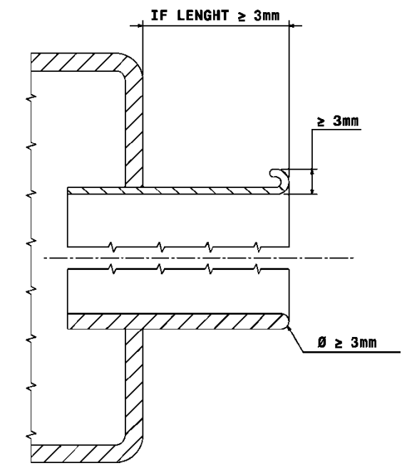
図6 サイレンサーの端部
