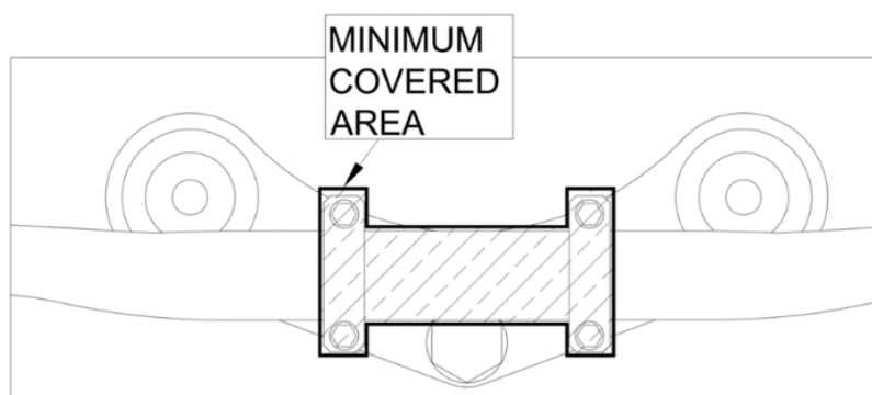
図2 ハンドルバーカバー
