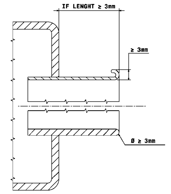
図6 サイレンサーの端部
