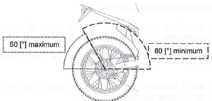
図 11 リアマッドガードの位置
