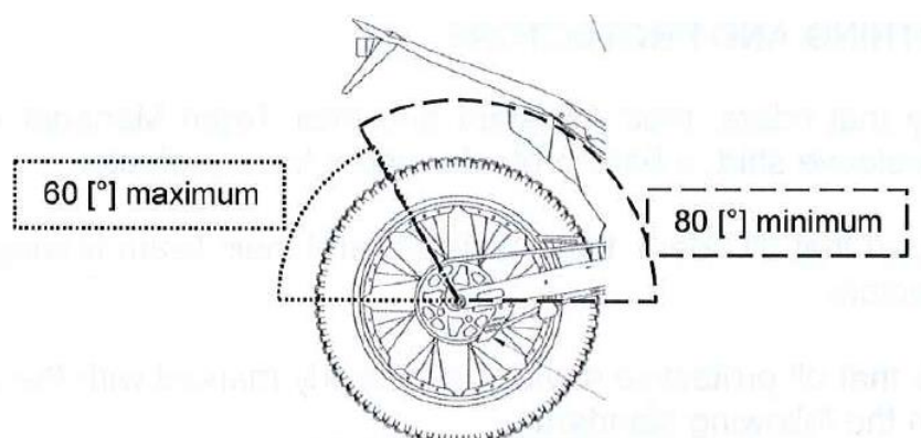
図 11 リアマッドガードの位置
